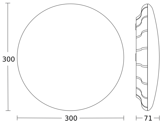
Disegno 1
